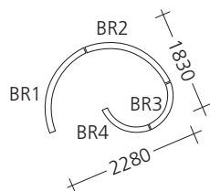
Abb. Bsp.4 Wandmodule komplett, Gesamtabmessung Breite x Tiefe 2280 x 1830mm
