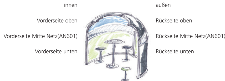
Abb. Bsp. 2 x Viertelkreis-Rundwand als Halbkreis
